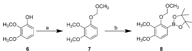
Scheme 1. (a) (i) NaH; (ii) ClCH 2 OCH 3 ; (b) (i) n -BuLi; (ii) 2-isopropoxy-4,4,5,5-tetramethyl-1,3,2-dioxaborolane.
